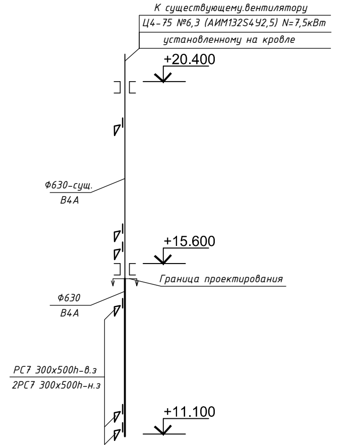
Фрагмент схемы системы В4А
