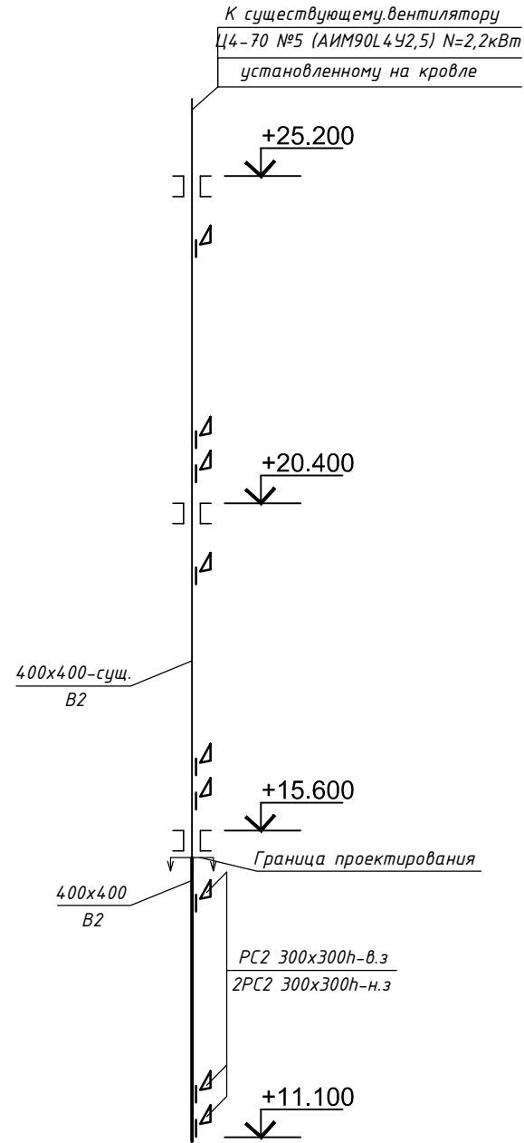
Фрагмент схемы системы В2
