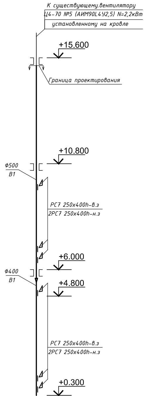
Фрагмент схемы системы В1
