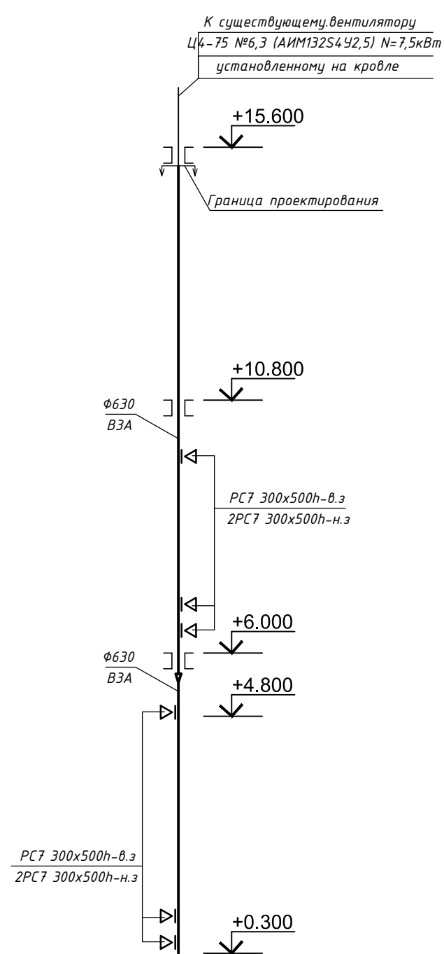
Фрагмент схемы системы В3А
